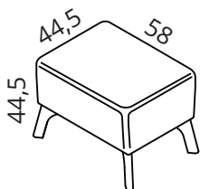
F1 Solid wood legs natural oak, wenge
